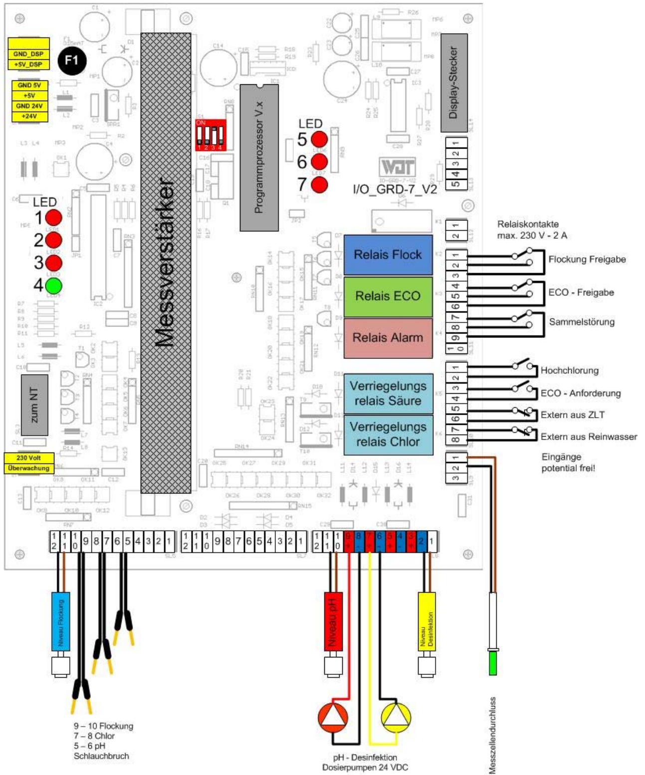
Die Abbildung zeigt die angeschlossenen Sensoren bzw. Verbraucher der Geräteversion 2S (mit zwei Schlauchpumpen).
